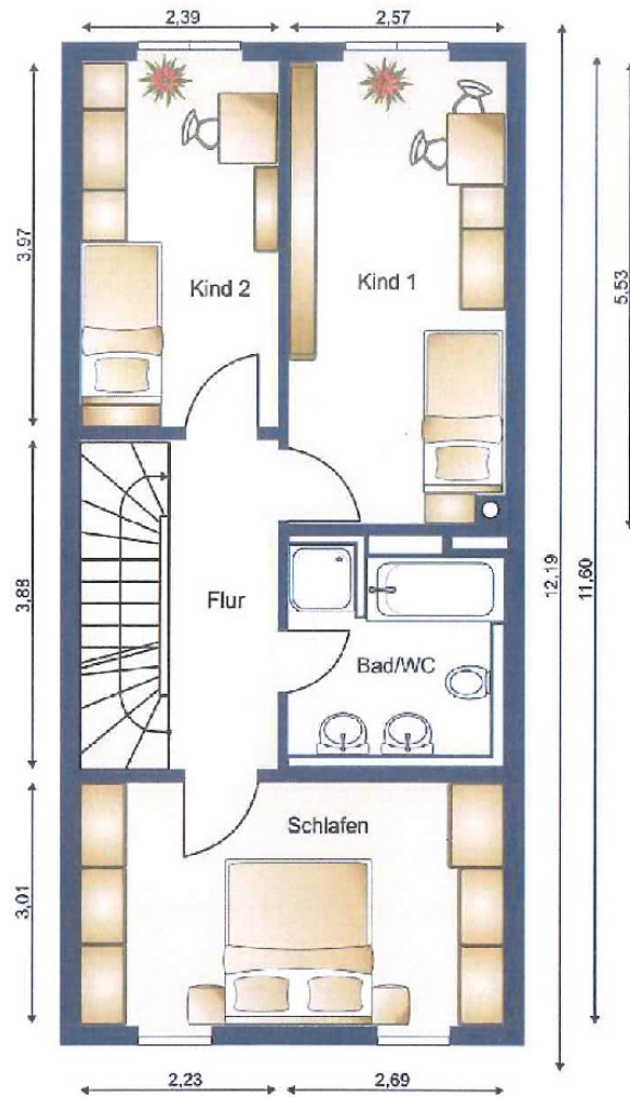
Grundriss Obergeschoss
