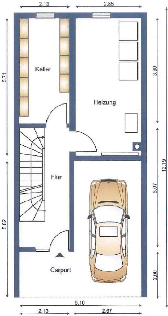
Grundriss Untergeschoss
