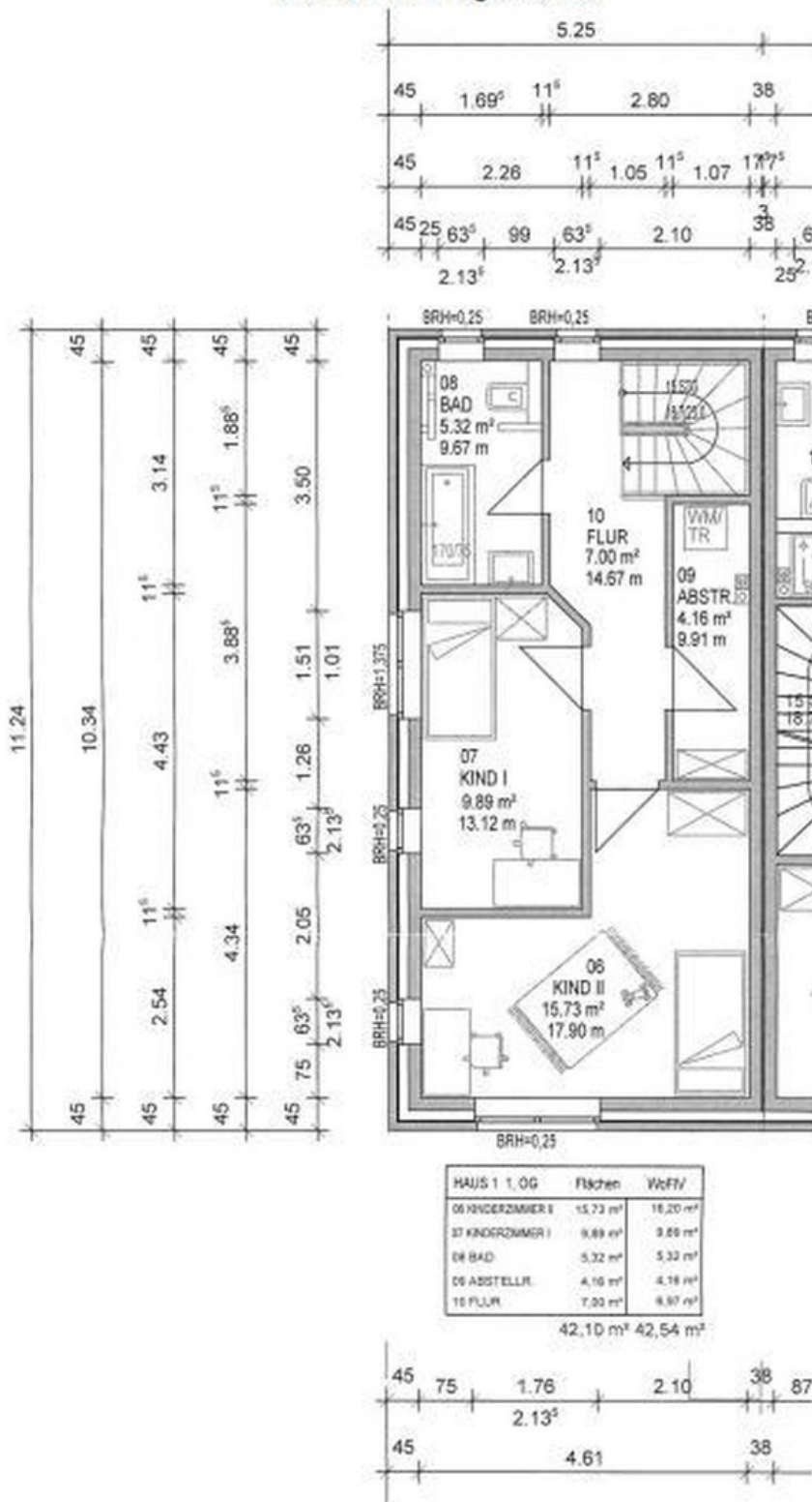
Grundriss Obergeschoss
