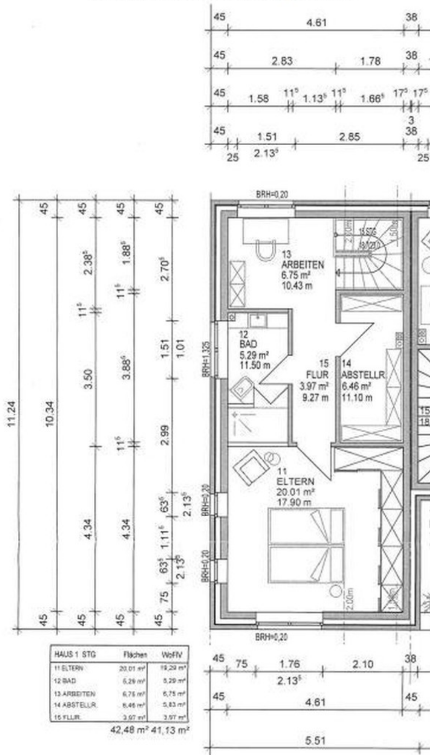
Grundriss Dachstudio/Staffelgeschoss
