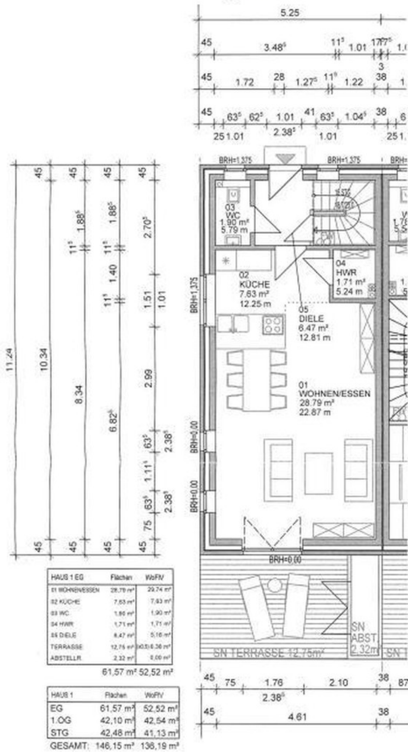
Grundriss Erdgeschoss
