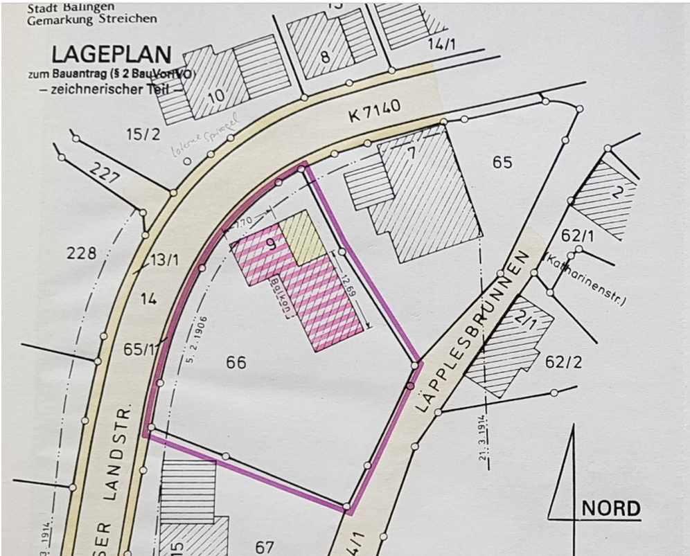
Lageplan
