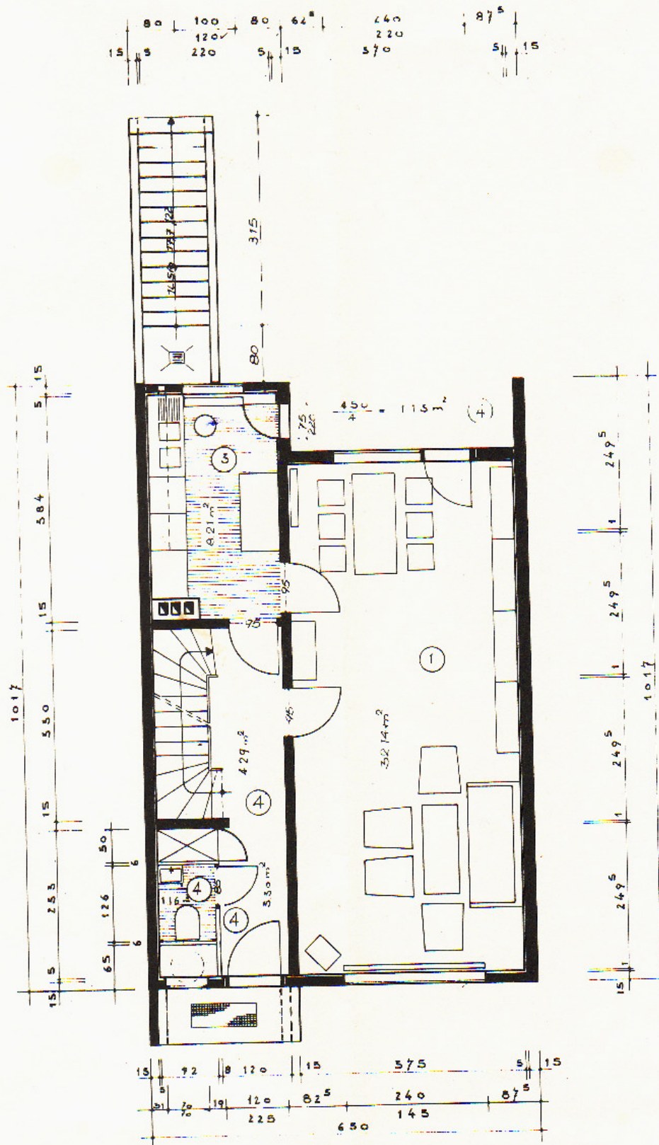
ERDGESCHOSS
