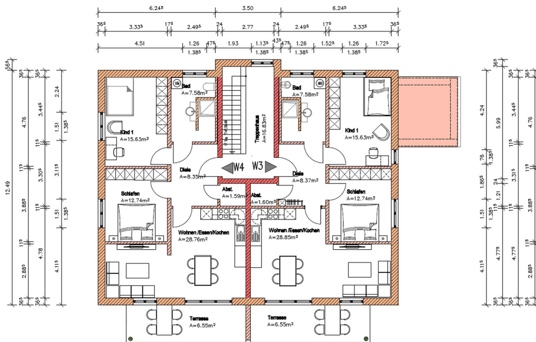
GRUNDRISS DG
