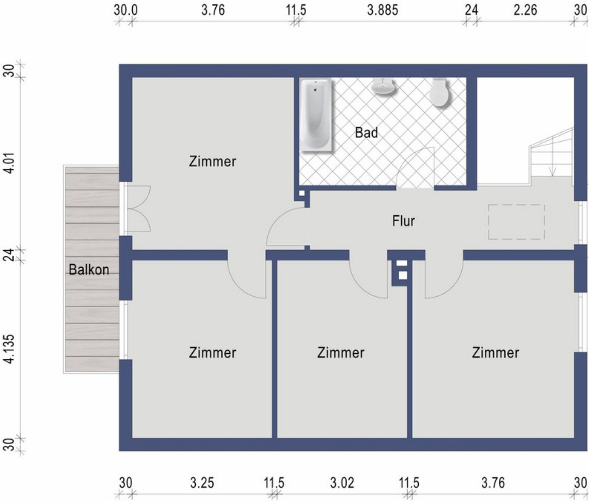
Obergeschoss
