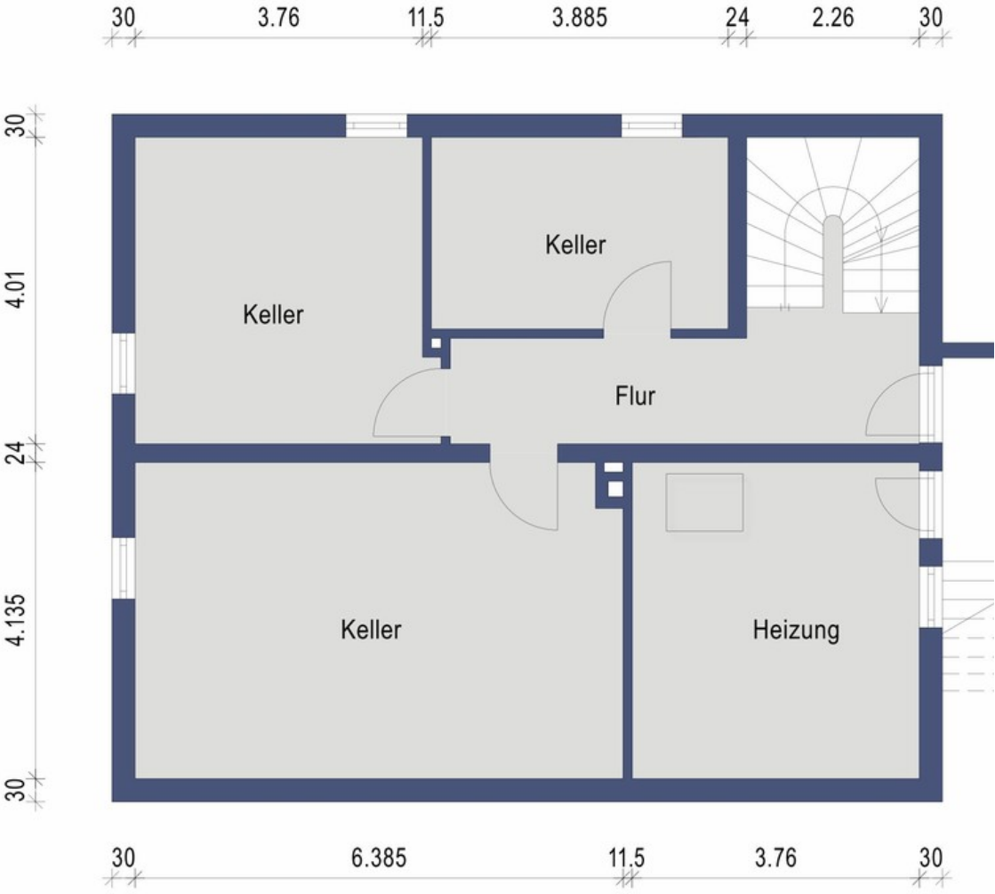
Kellergeschoss
