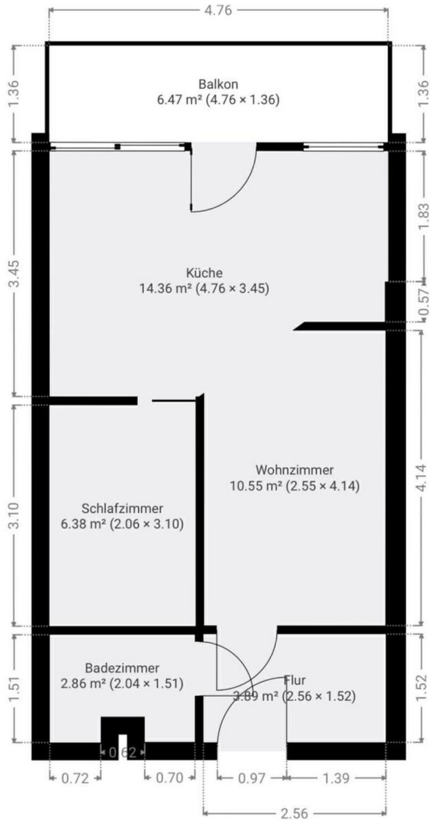
Grundriss
