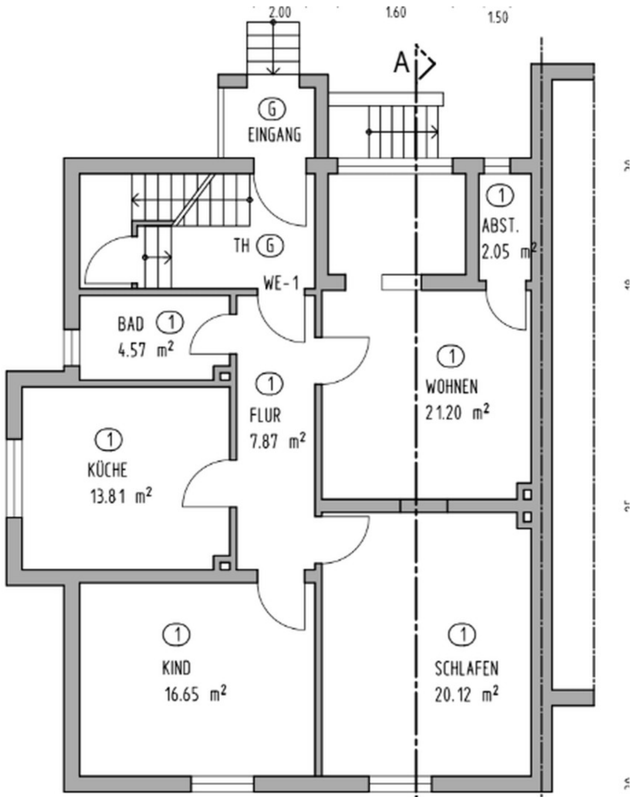
Grundriss
