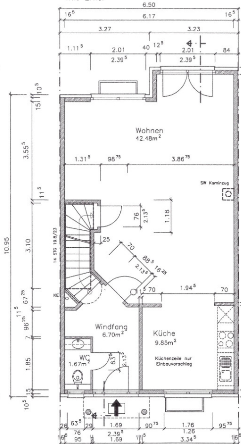
ERDGESCHOSS mit Erker
