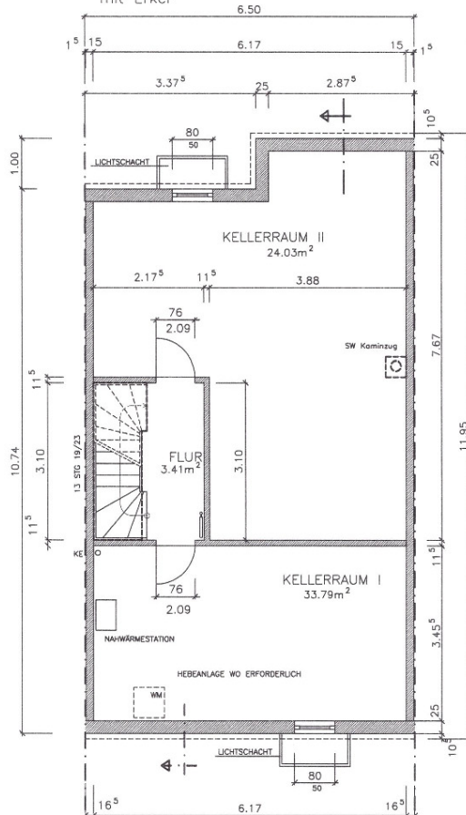
KELLERGECHOSS mit Erker
