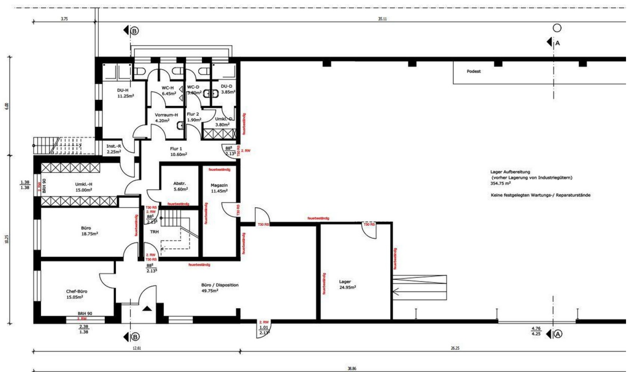
Gebäude Erdgeschoss
