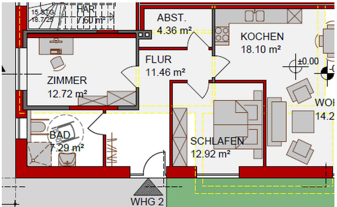
Grundriss Wohnung 2
