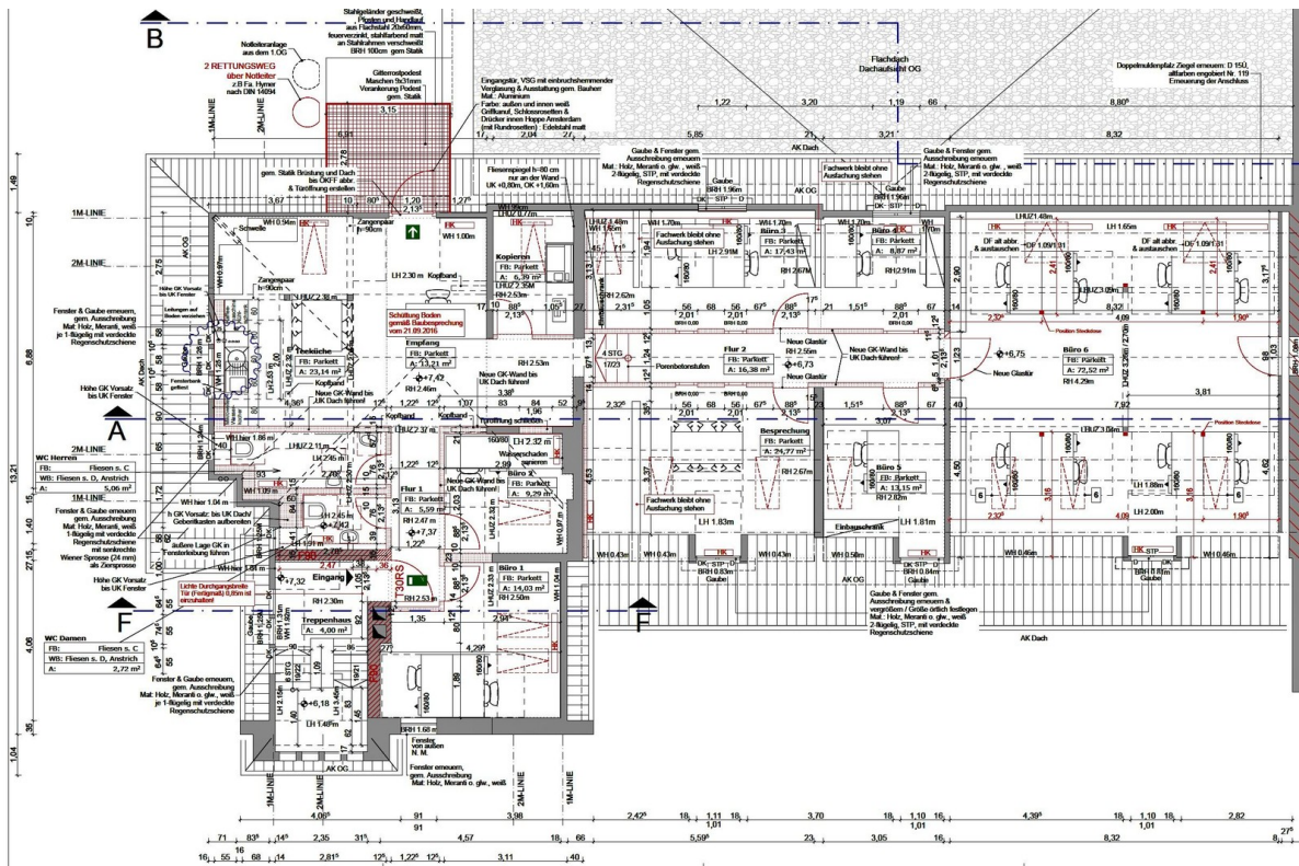
Grundriss
