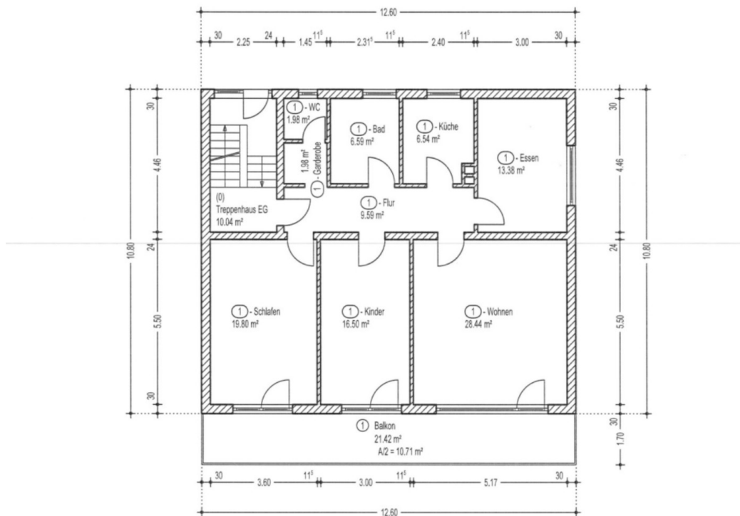
Grundriss
