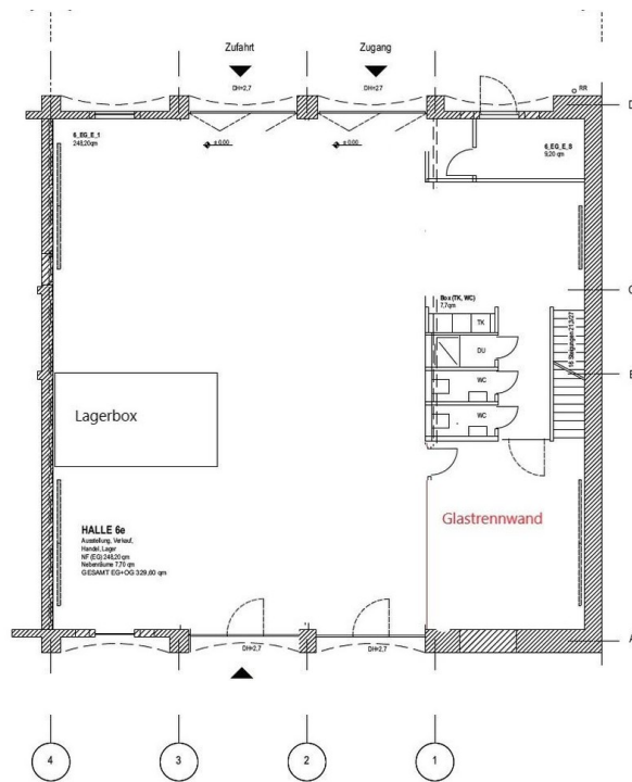
HALLE 6E Grundriss EG
