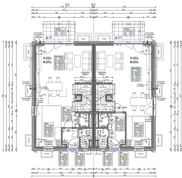
Grundriss Erdgeschoss
