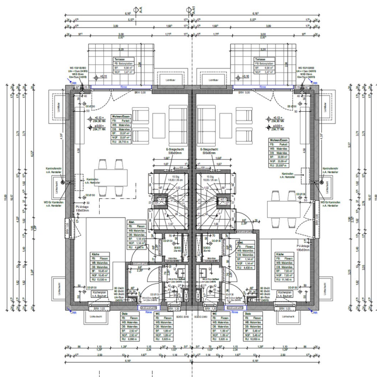
Grundriss Erdgeschoss
