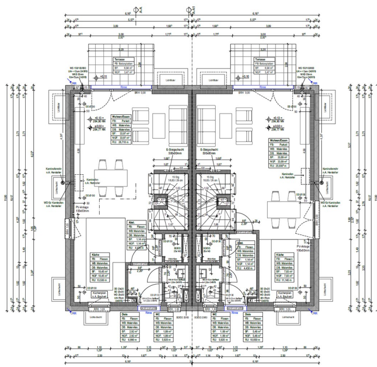
Grundriss Erdgeschoss
