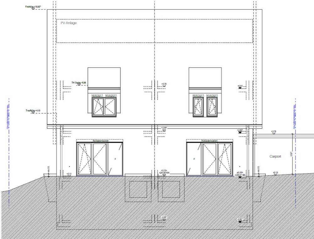
Gartenansicht
