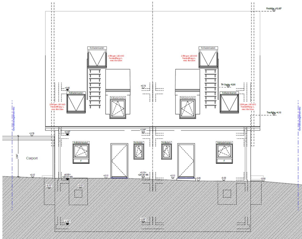
Straßenansicht
