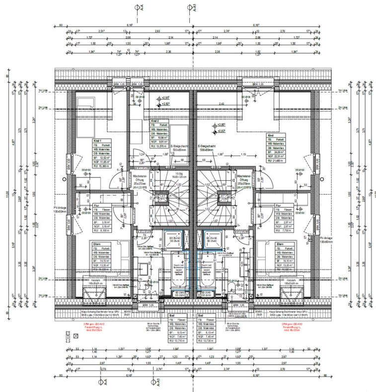
Grundriss Dachgeschoss
