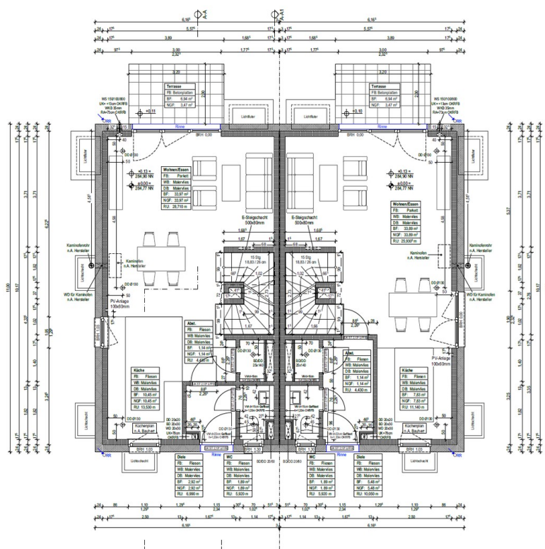
Grundriss Erdgeschoss
