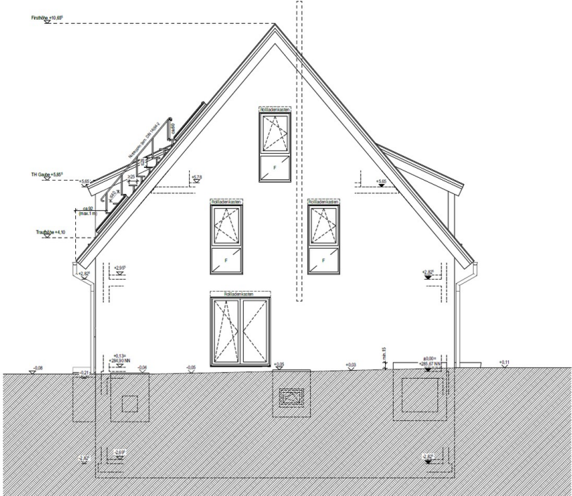
Seitenansicht
