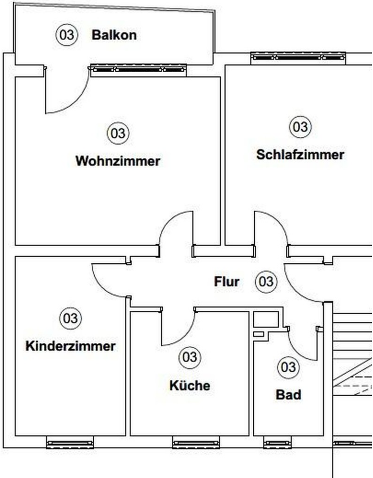
Grundriss
