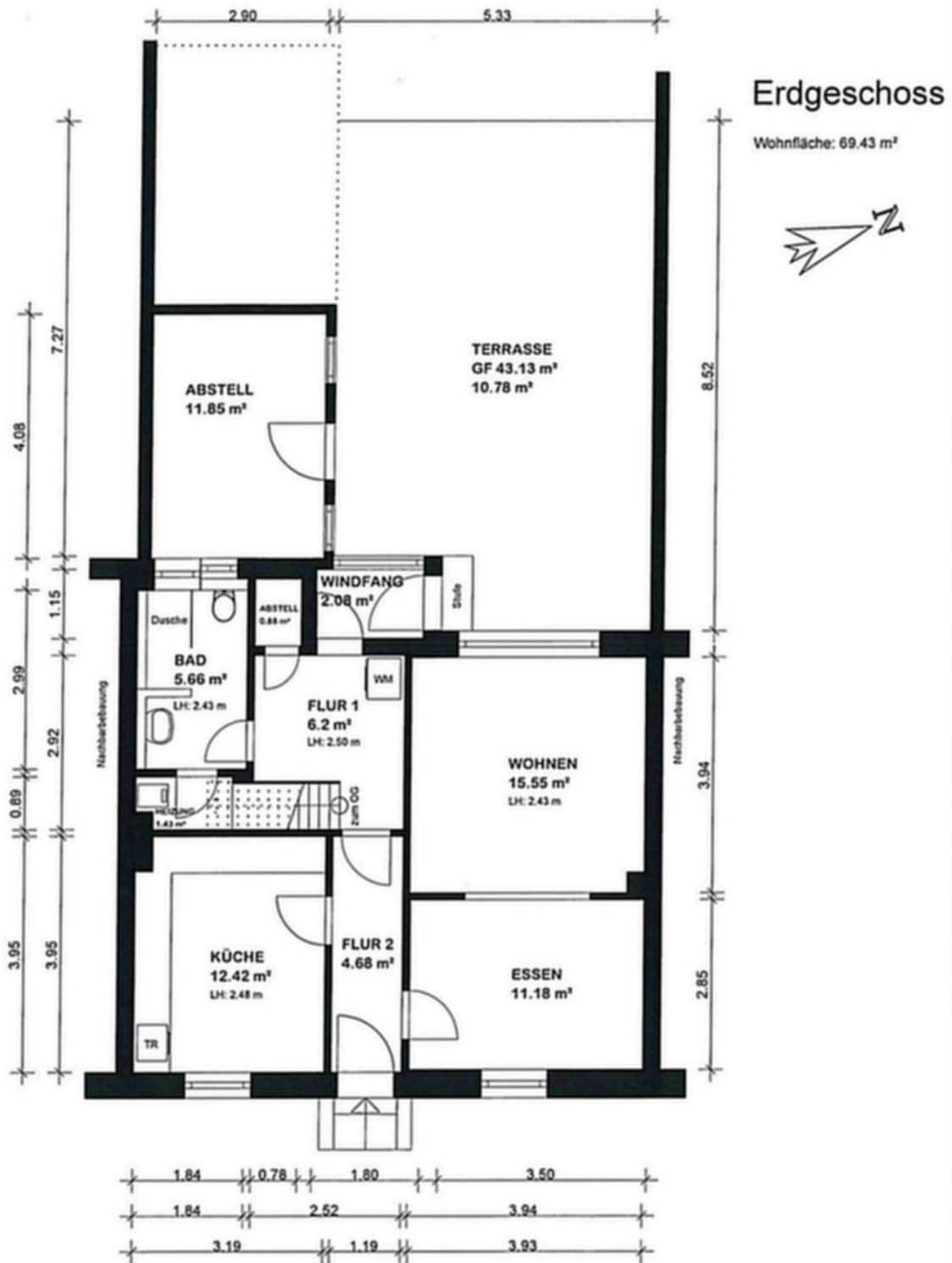
Grundriss EG
