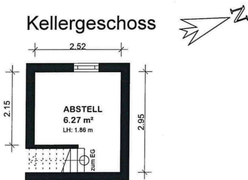
Grundriss Keller
