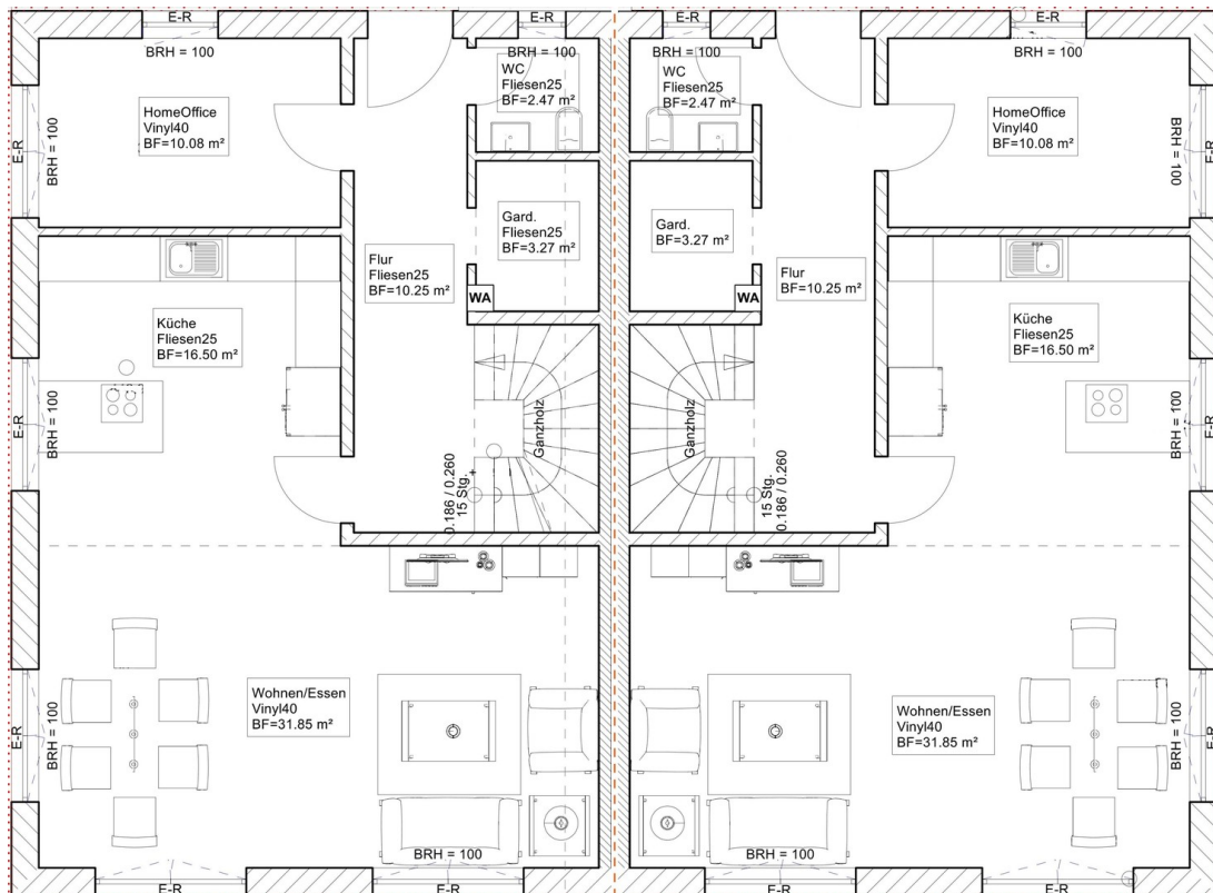
Erdgeschoss
