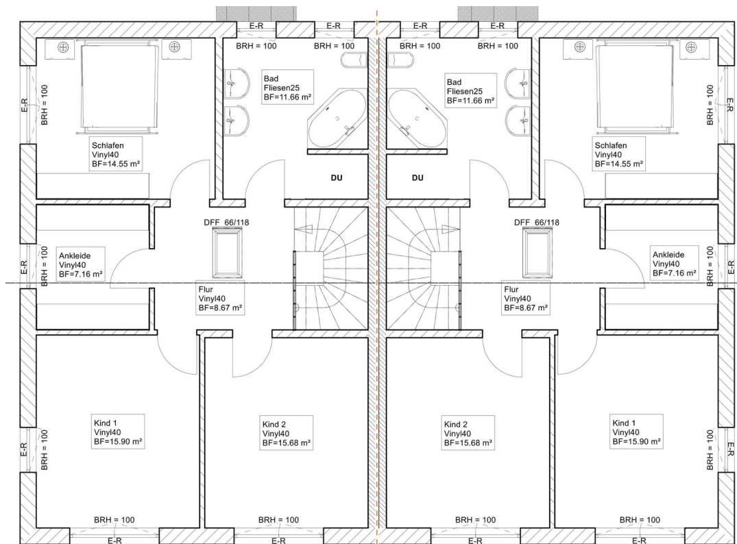
Dachgeschoss
