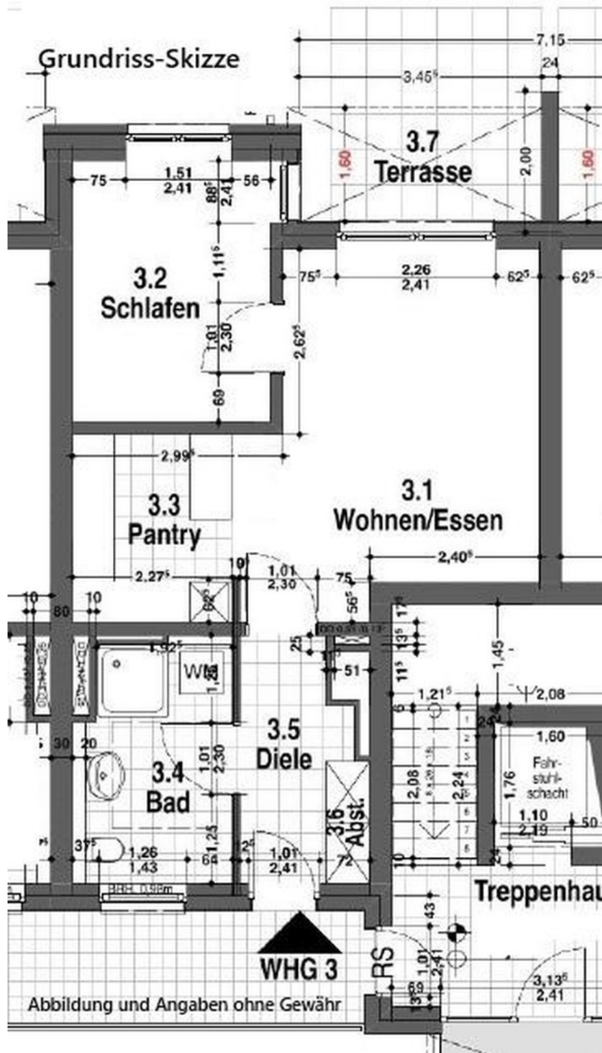
Grundriss-Skizze
