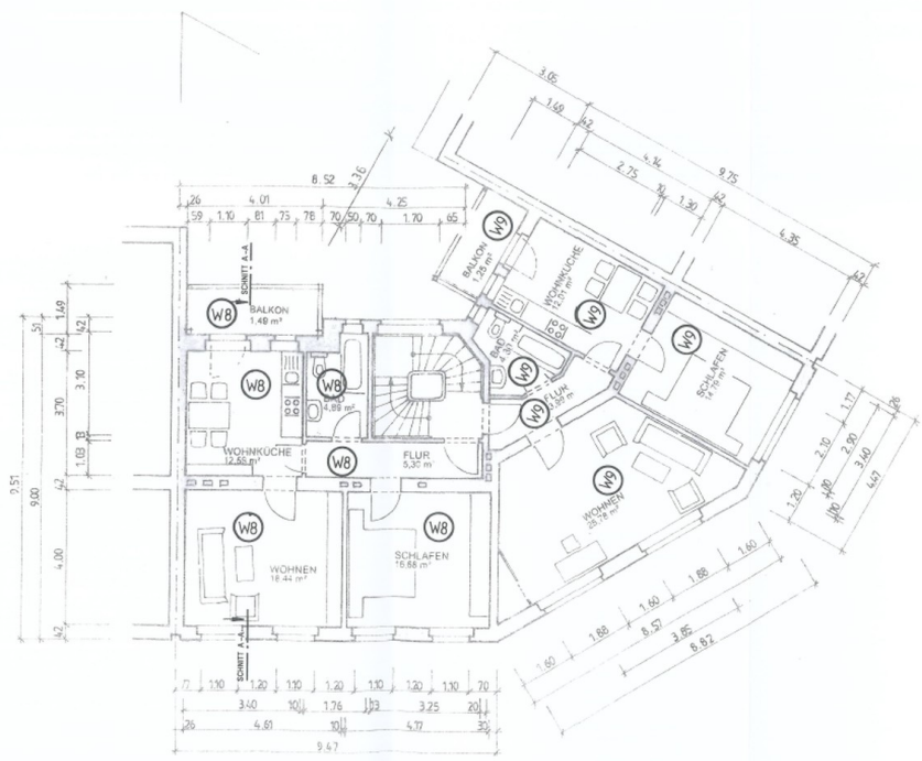
4. OBERGESCHOSS
