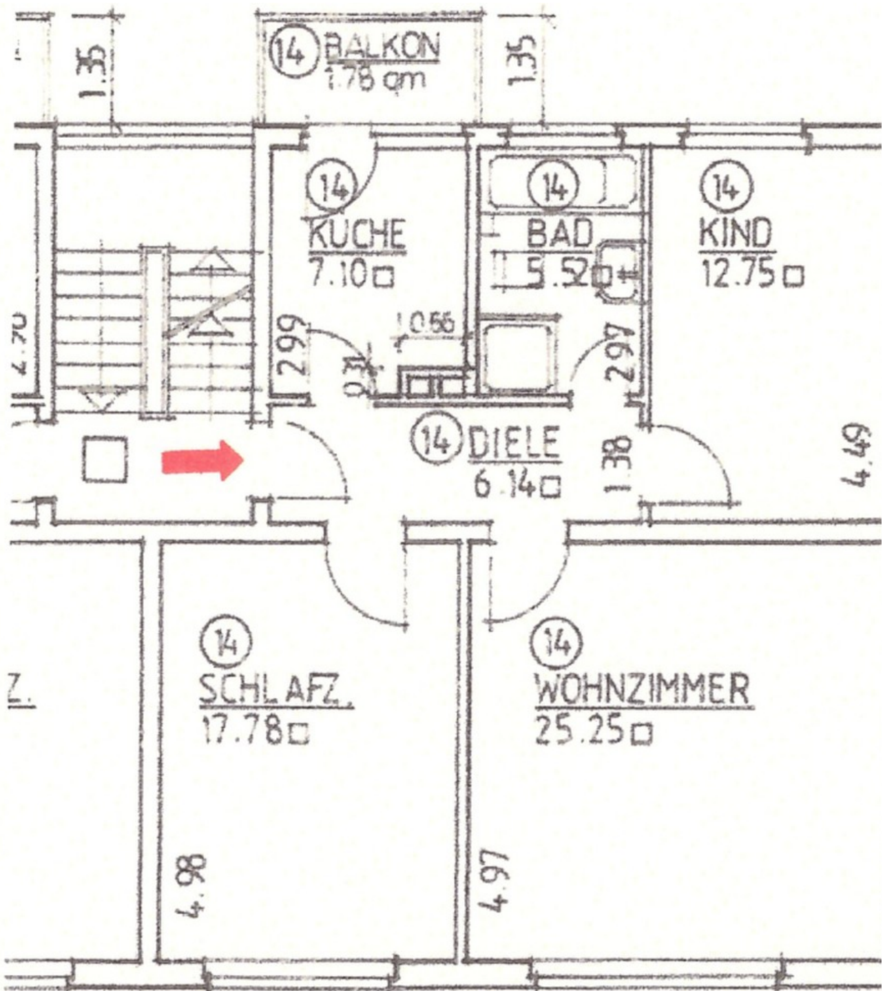
2. Obergeschoss (Wohnung Nr. 14)
