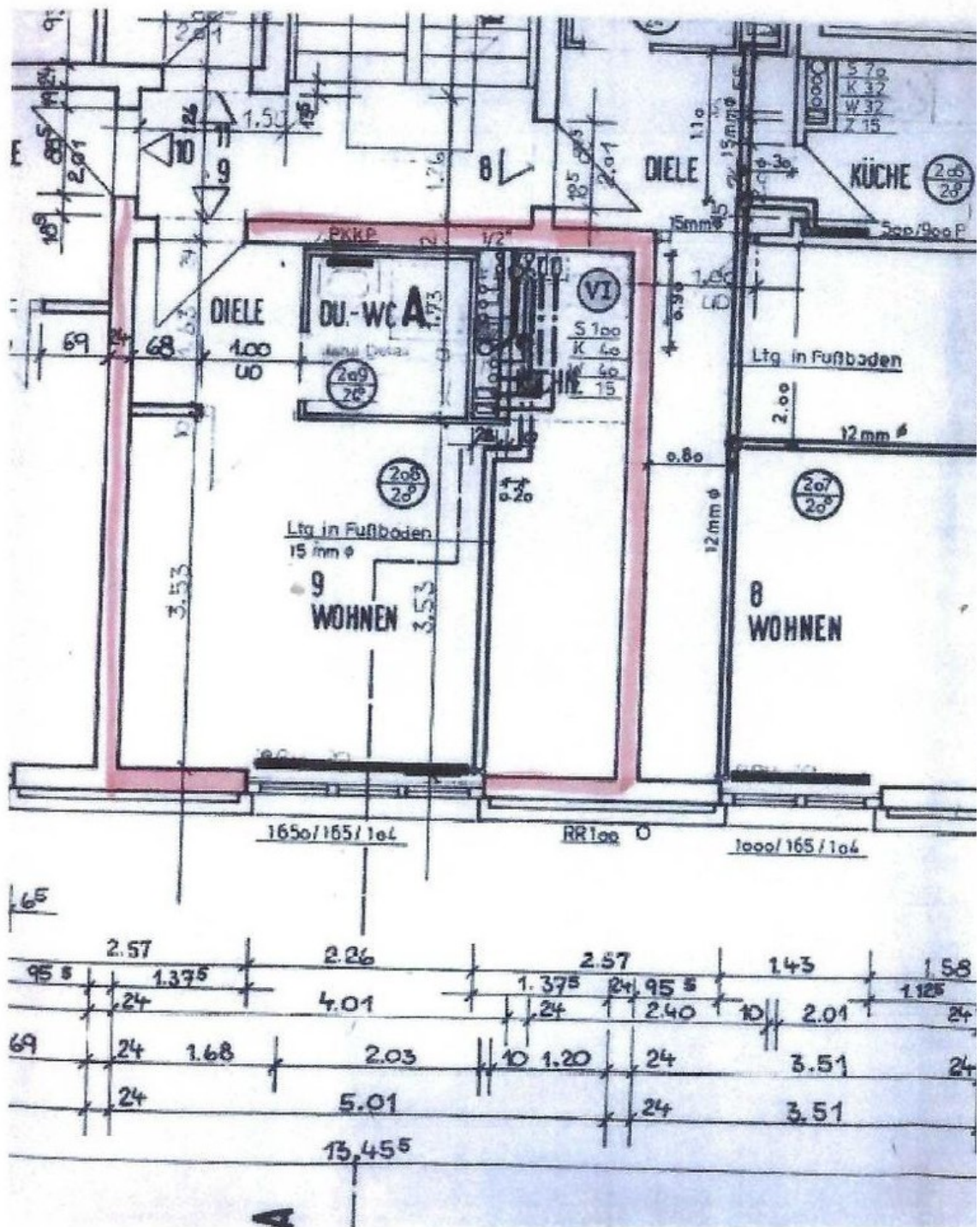
Grundriss
