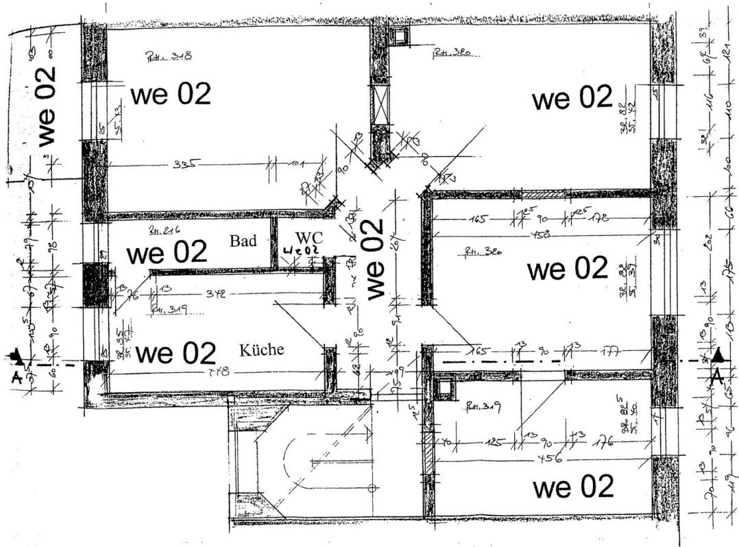
Grundriss
