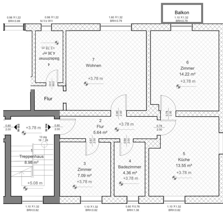
Grundriss Wohnung rechts
