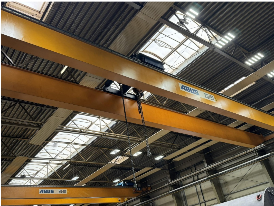
Krananlagen
