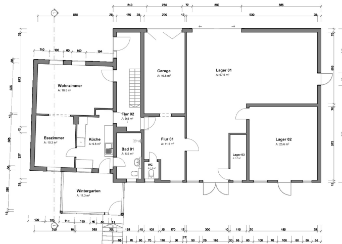
Erdgeschoss 1:100
