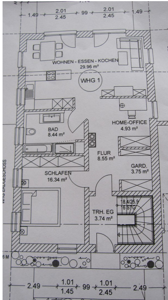
Grundriss
