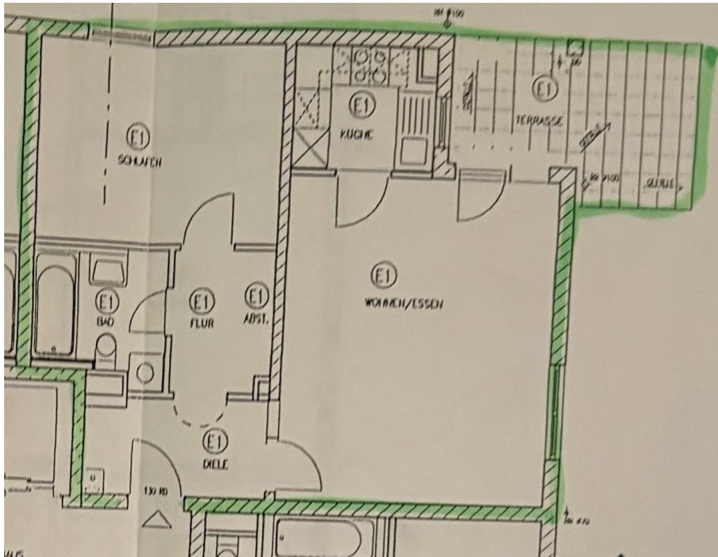
Grundriss Wohnung
