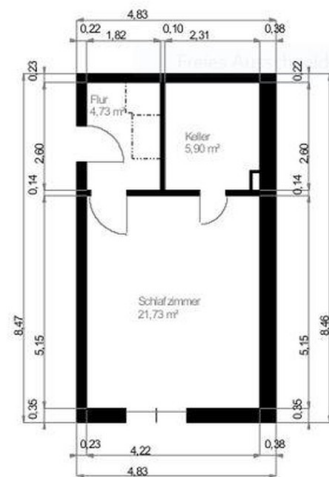
Grundriss Souterrain
