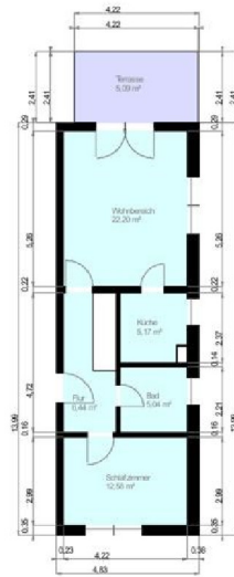
Grundriss EG
