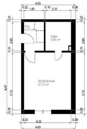
Grundriss Souterrain
