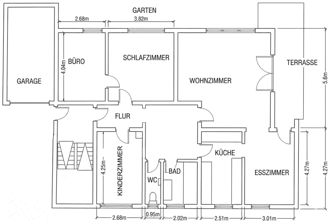
Grundriss
