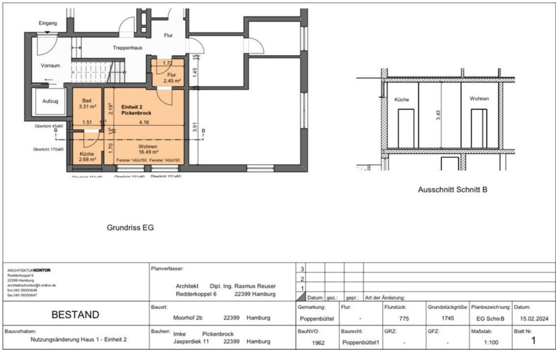
Grundriss
