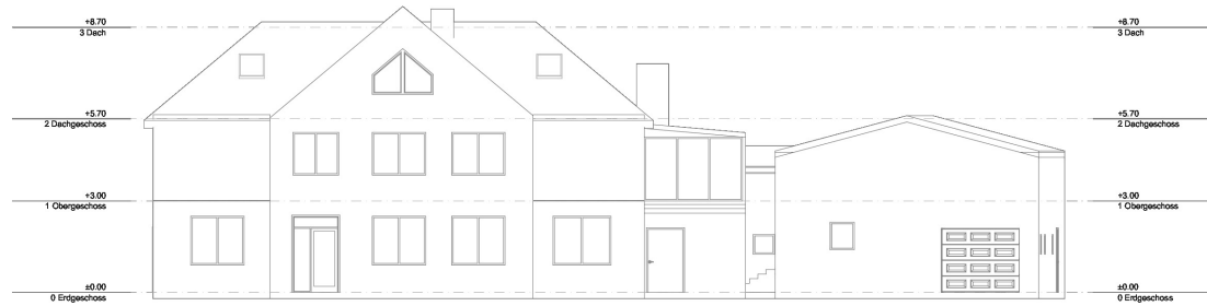
Südansicht 1:100
