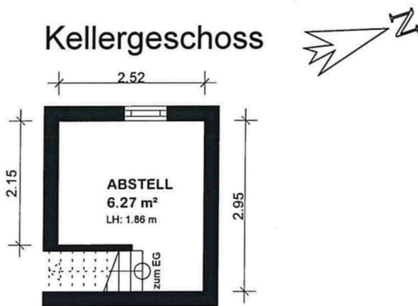
Grundriss Keller
