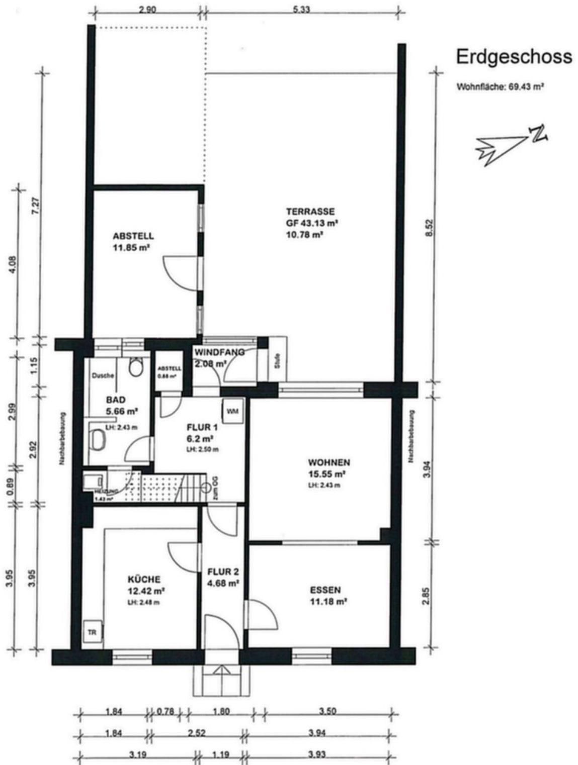
Grundriss EG
