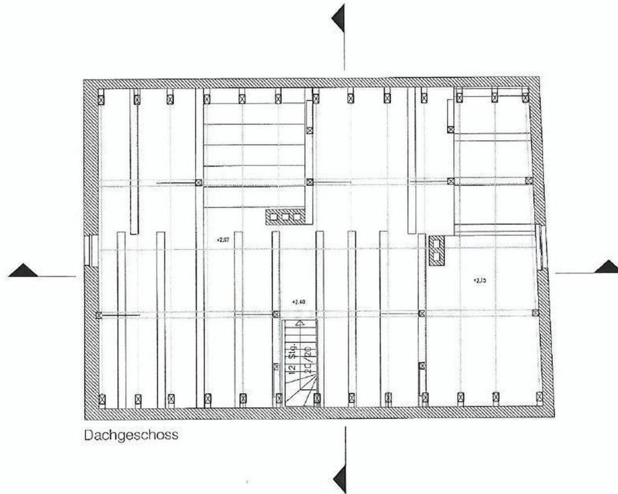
Dachgeschoss
