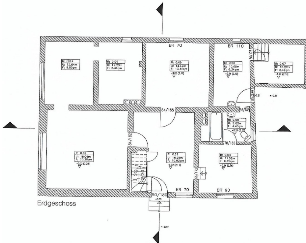
EG - momentaner Grundriss
