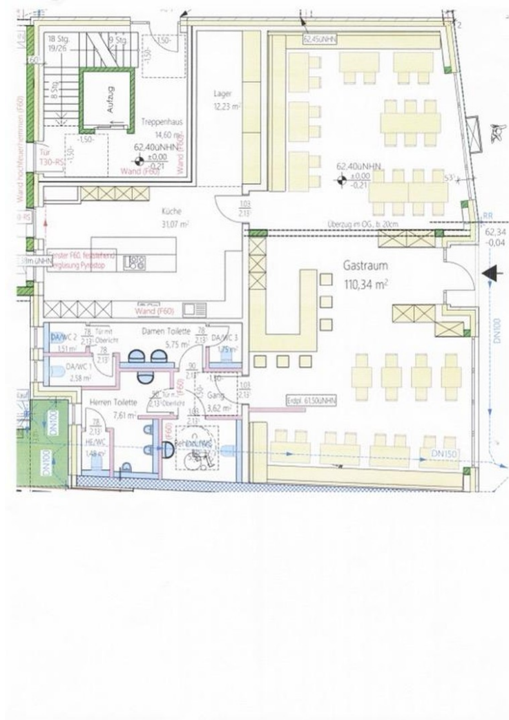
Exemplarischer Grundriss
