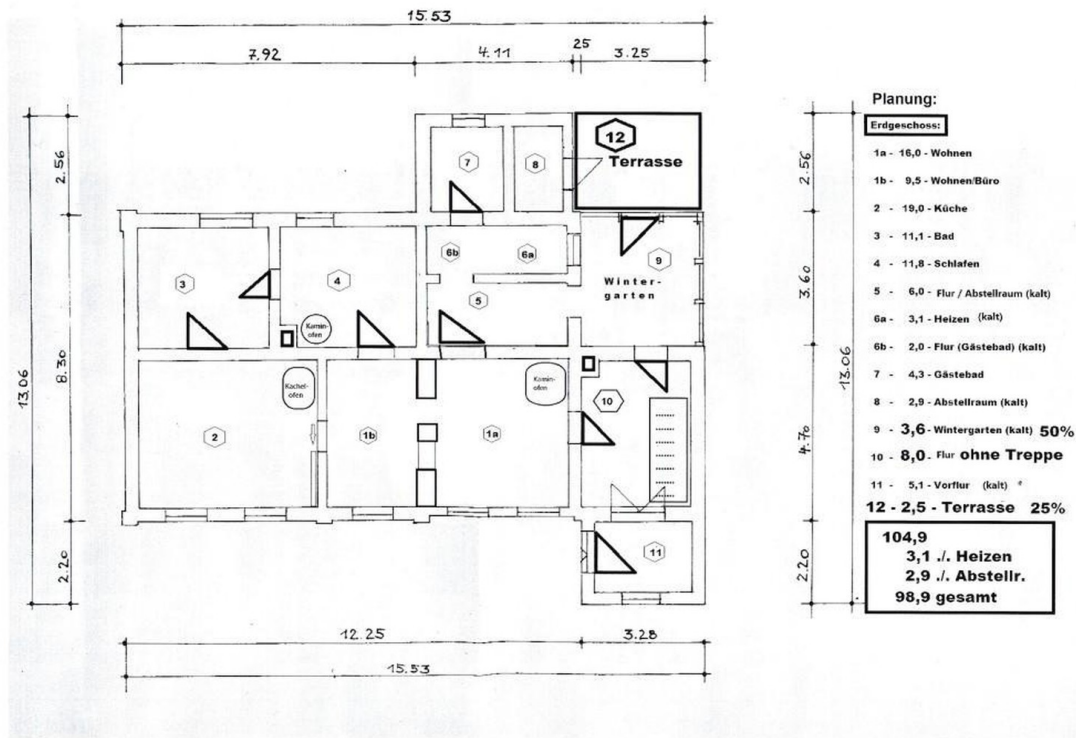
Planung Erdgeschoss
