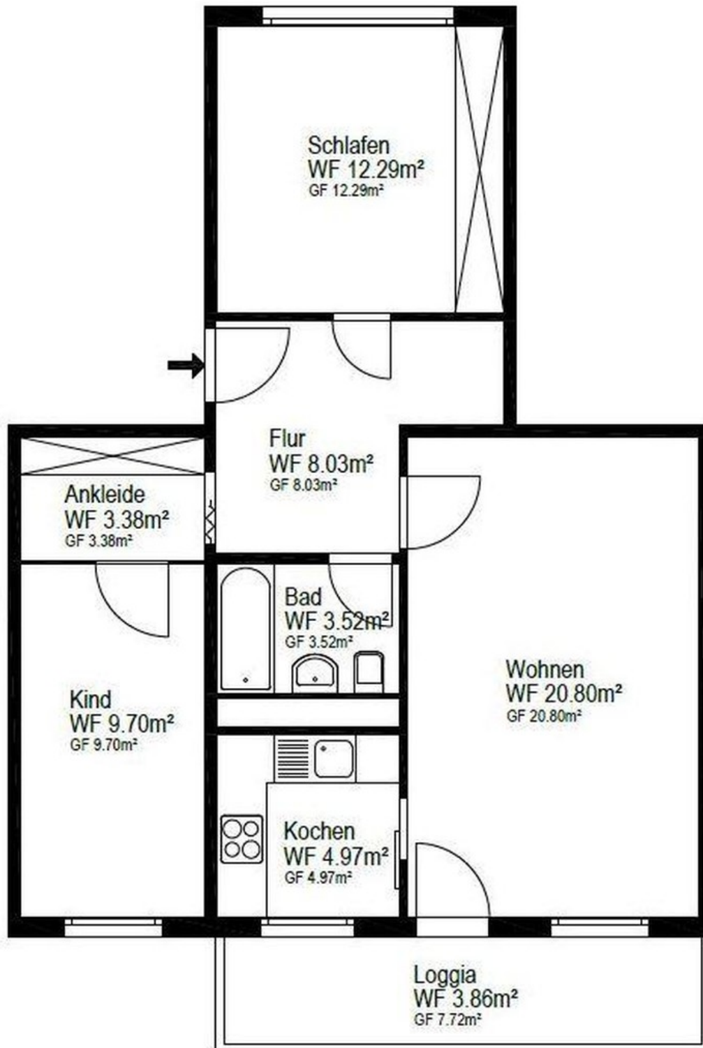
Grundriss
