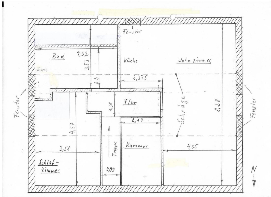
Grundriss Dachgeschoss
