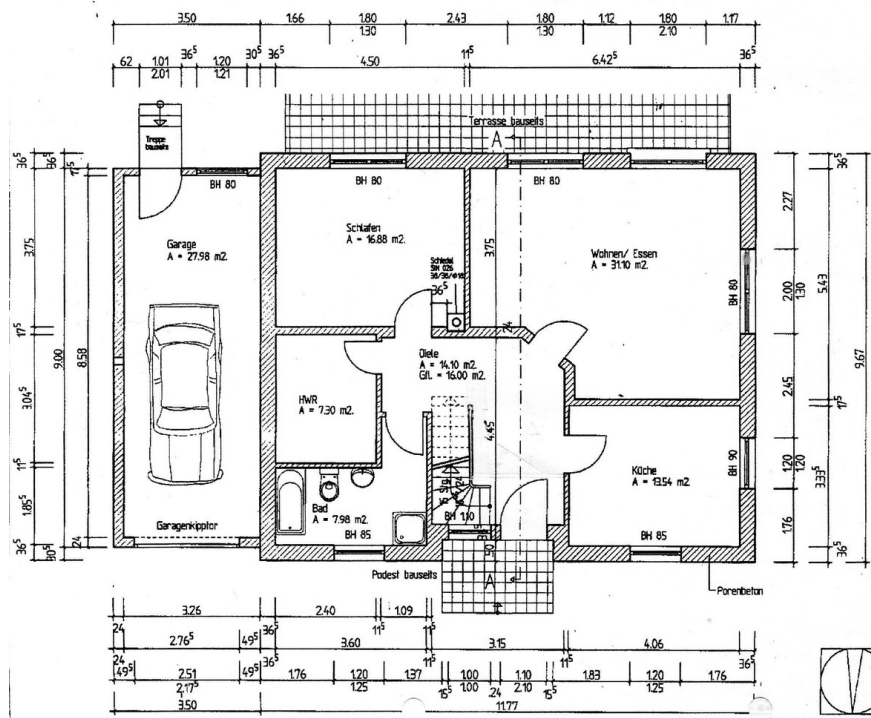
Grundriss Erdgeschoss
