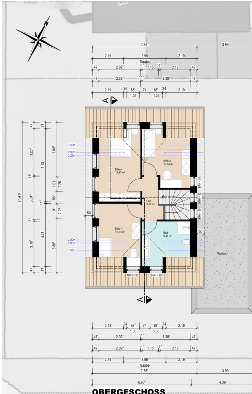
Grundriss Obergeschoss
