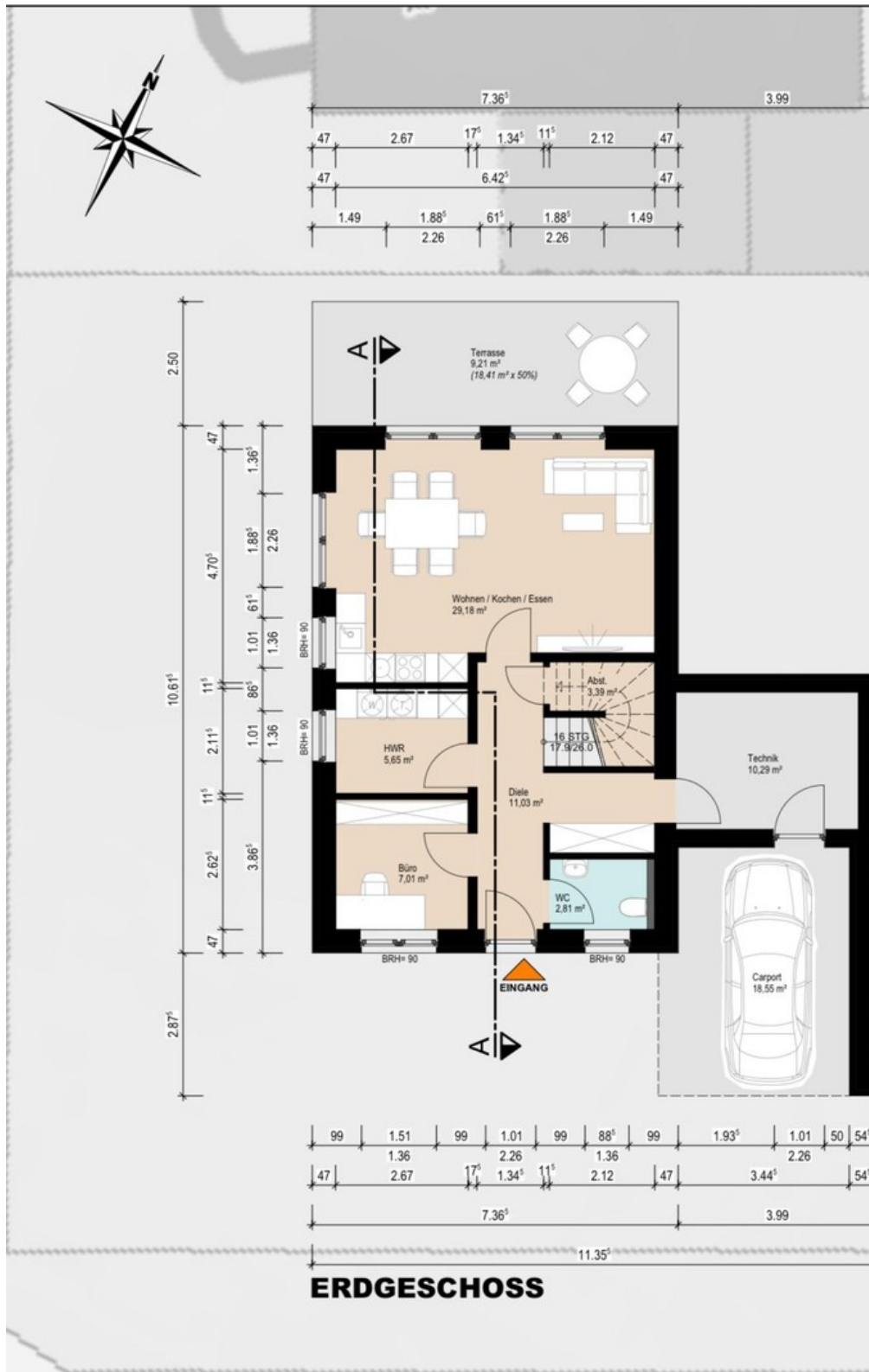
Grundriss Erdgeschoss
