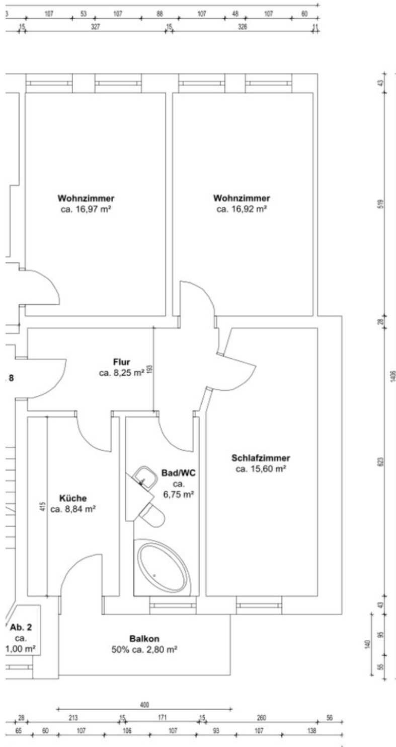
Grundriss
