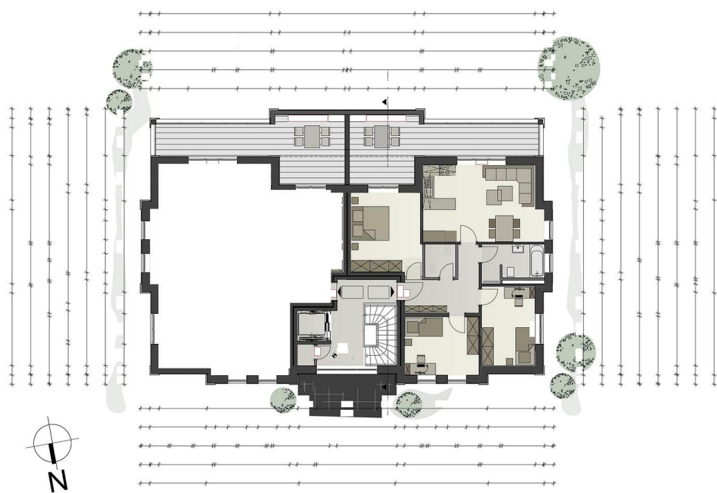
GRUNDRISS 1.OBERGESCHOSS
