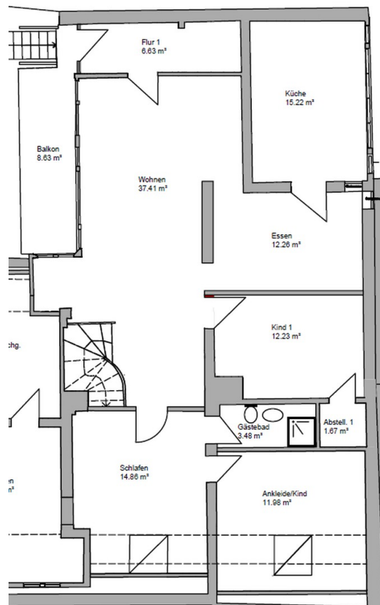
Grundriss unten
