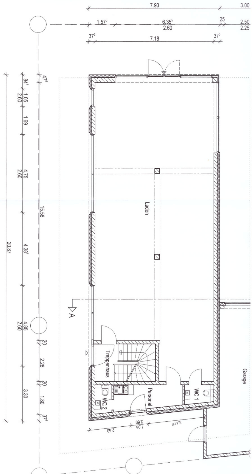
Grundriss Erdgeschoss
