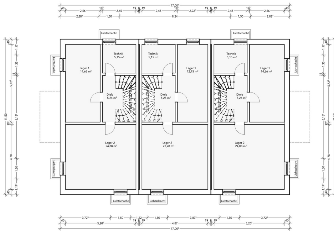
Grundriss Untergeschoss
