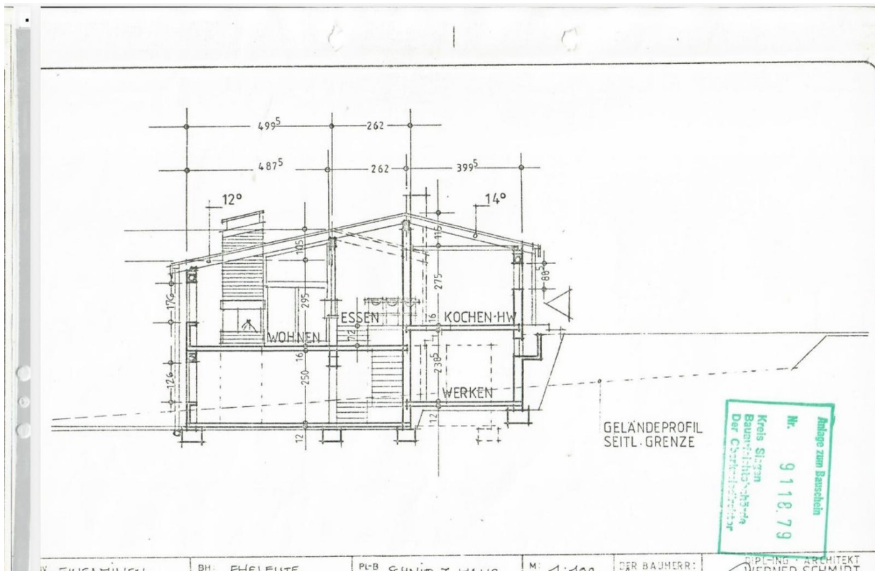
Schnitt
