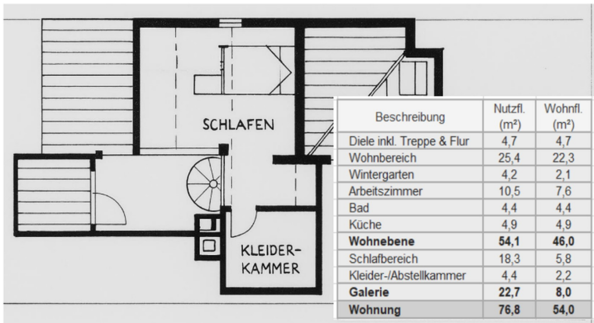
Grundriss Obergeschoss (4. OG)
