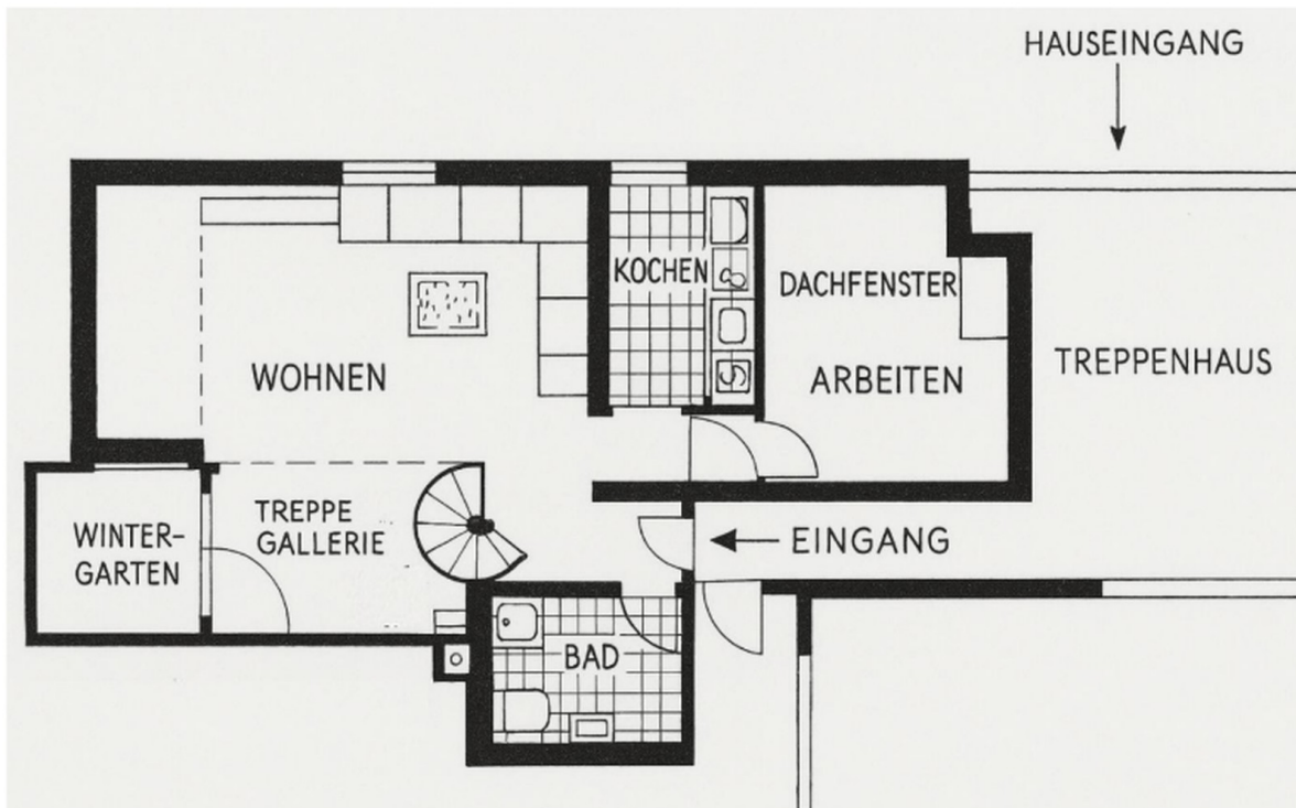
Grundriss (3. OG)
