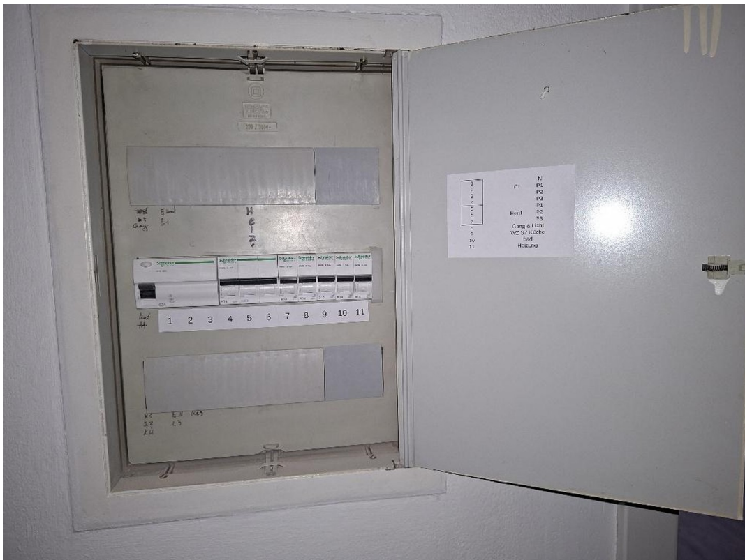
Sicherungskasten mit FI
